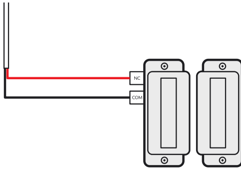
Door Position Sensor
