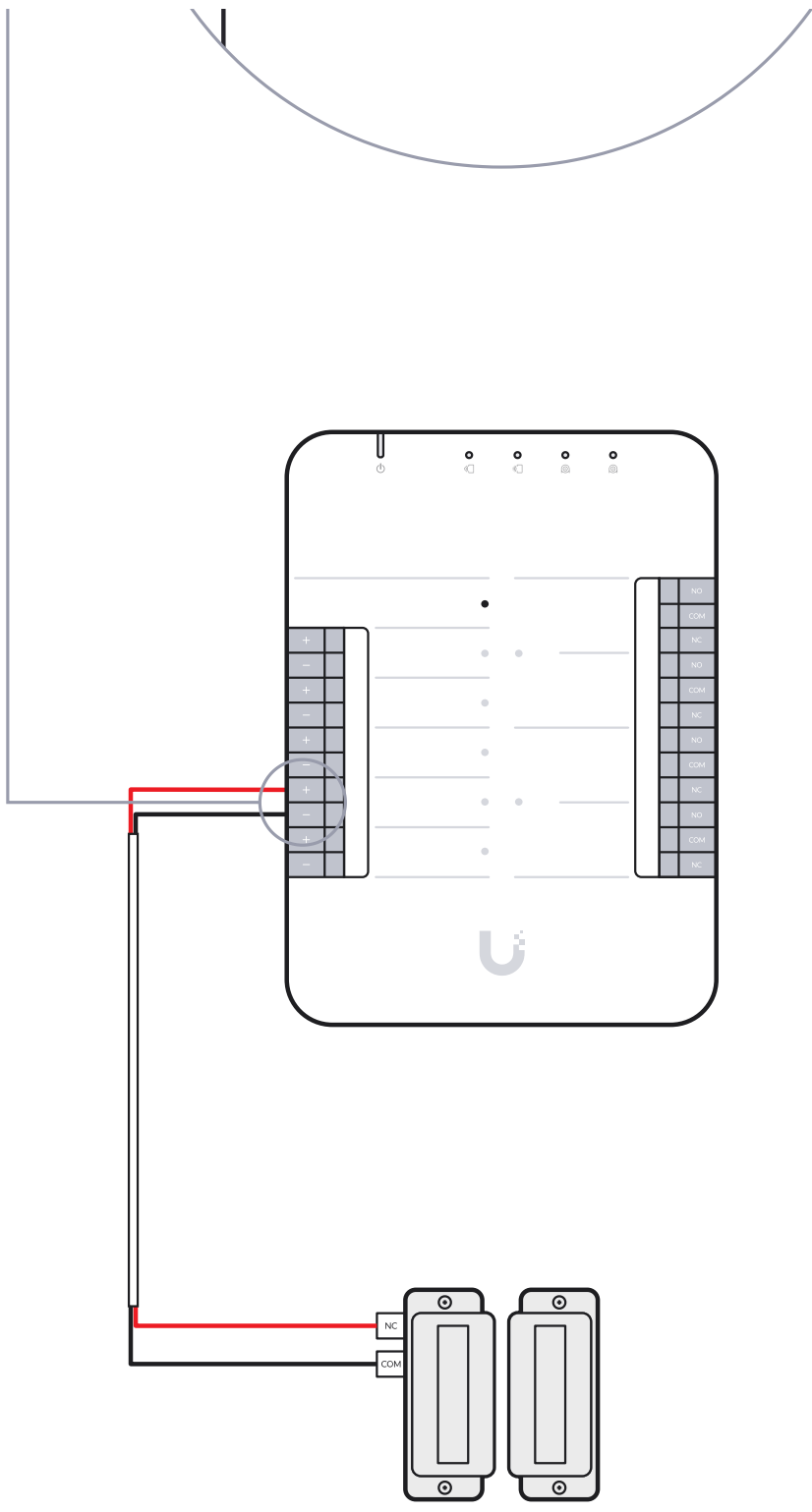
Door Position Sensor
